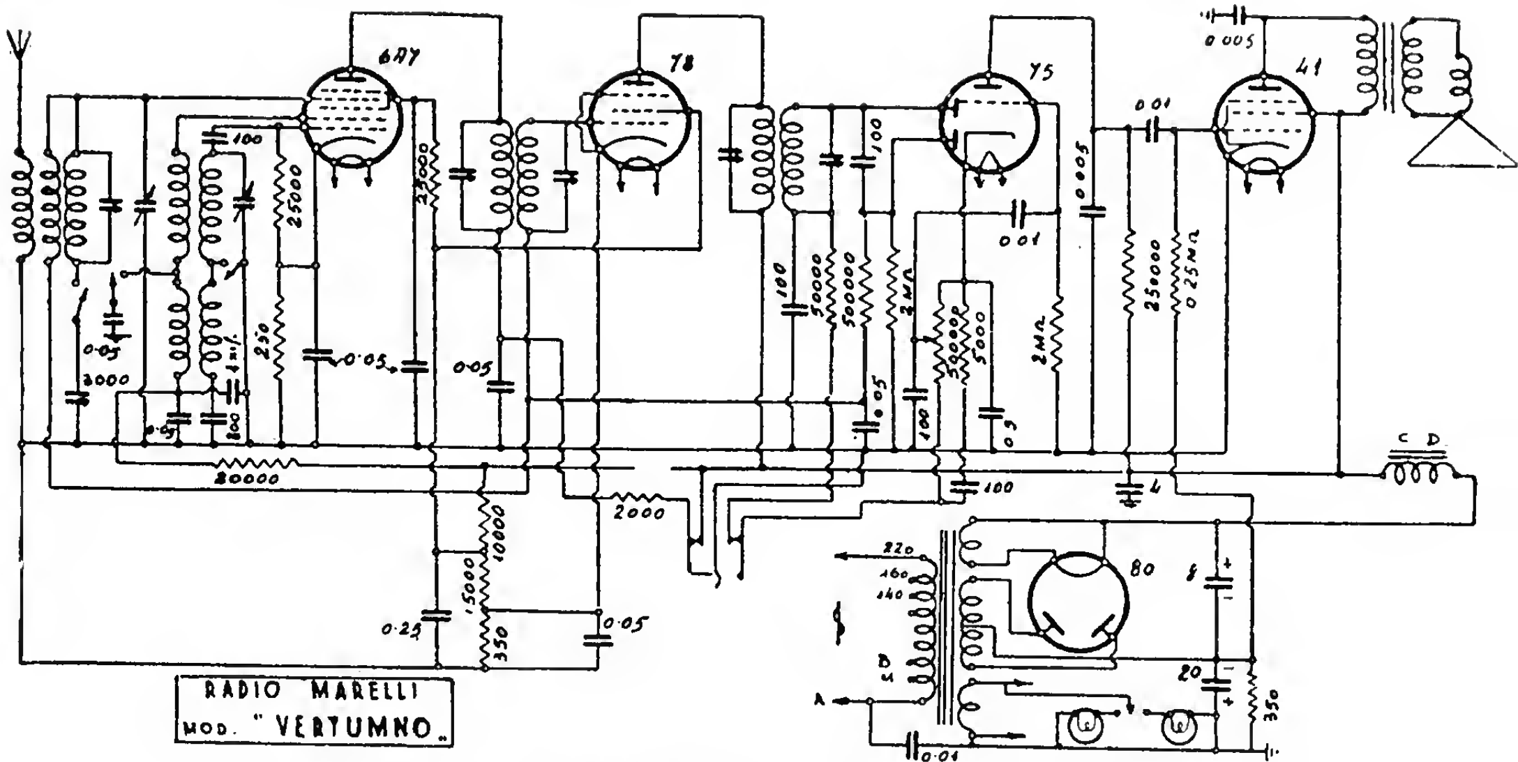
RADIO MARELLI — Modello « Vertumno ». - Produzione 1934. - Media frequenza: 485 kc.
