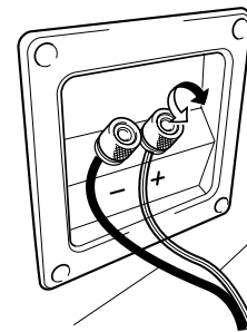
ライン無しのコード ステレオアンプのスピーカー出力端子の⊖へ
